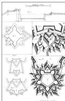
Fortifikaciniai statiniai: Encyclopédie (Art militaire, fortifications, planche IV)
